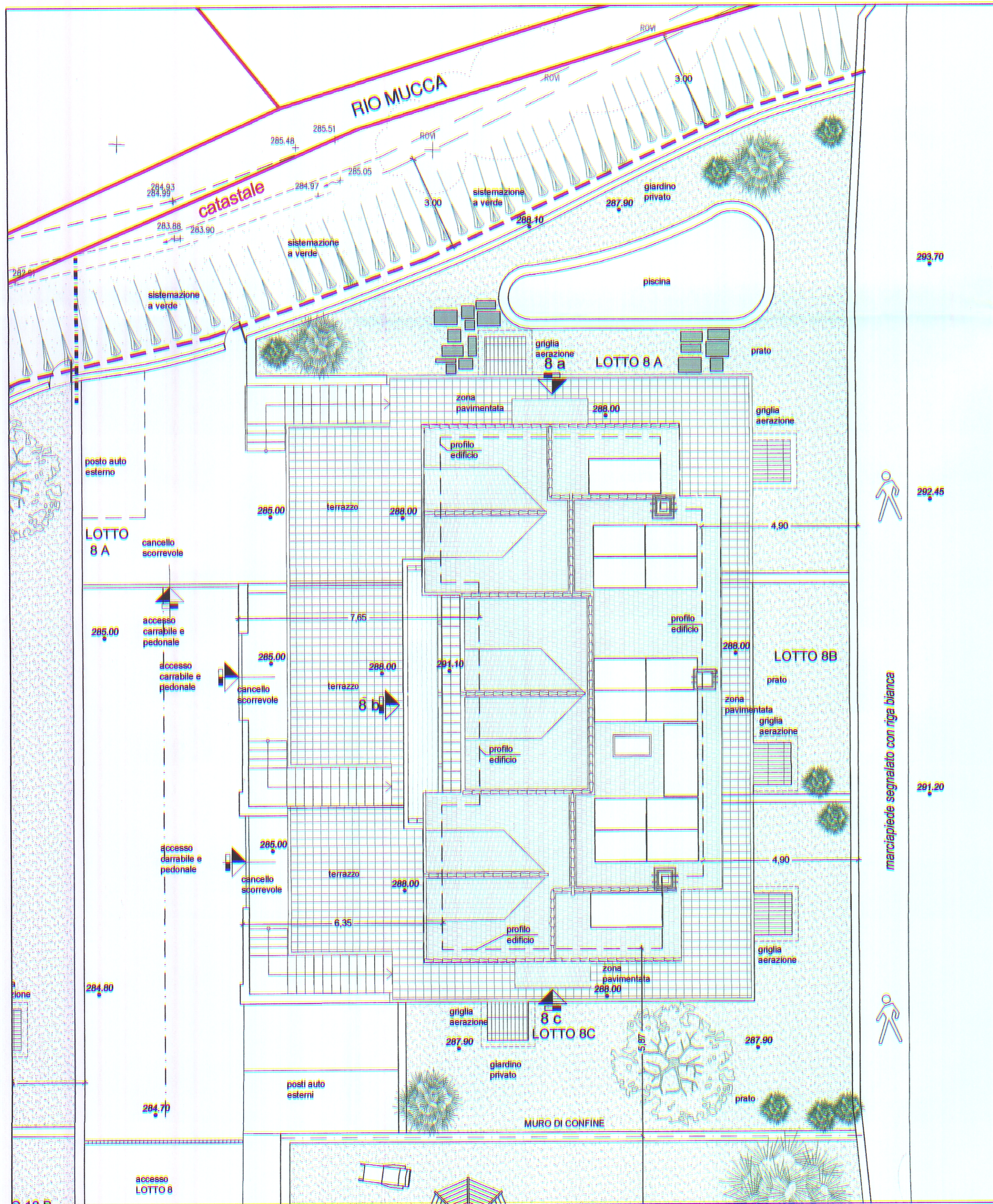
PLANIMETRIA _scala 1:100
