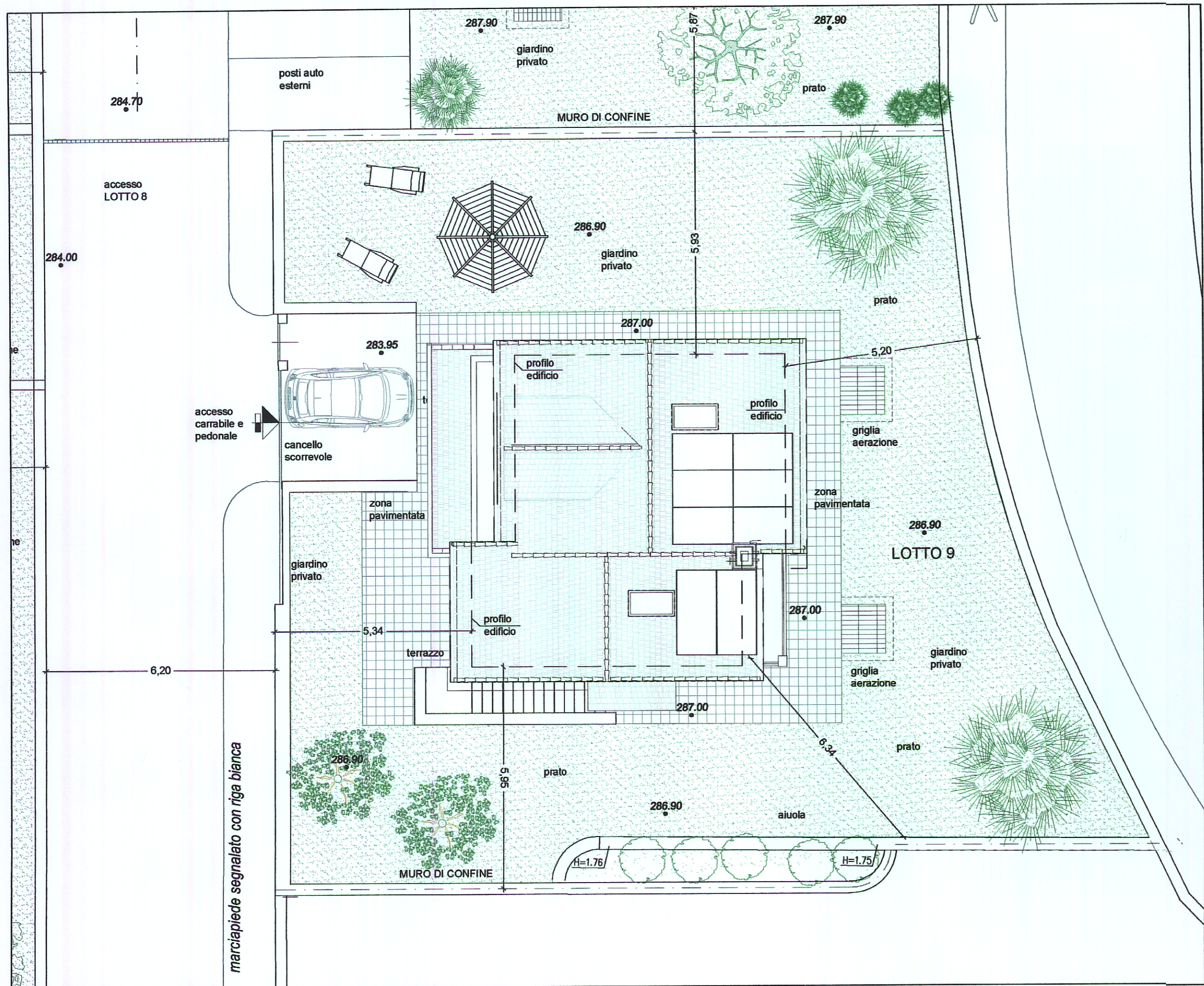
PLANIMETRIA _scala 1:100
