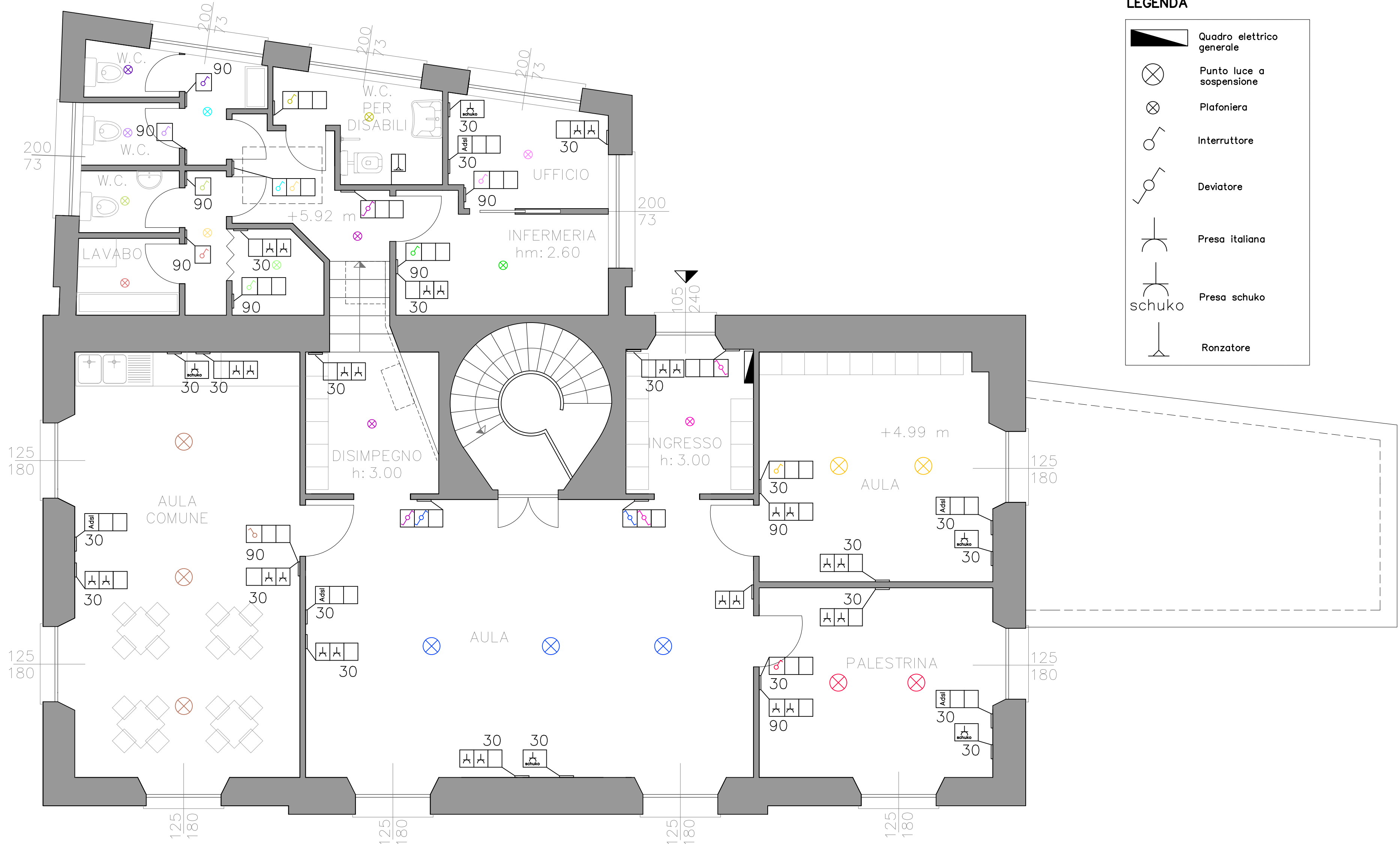
PIANTA PIANO PRIMO – sezione +6.20 m Scala 1:50
