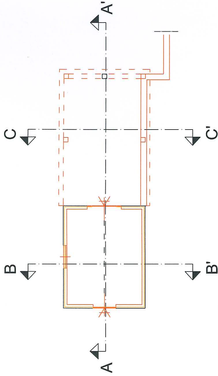
- PIANTA -
