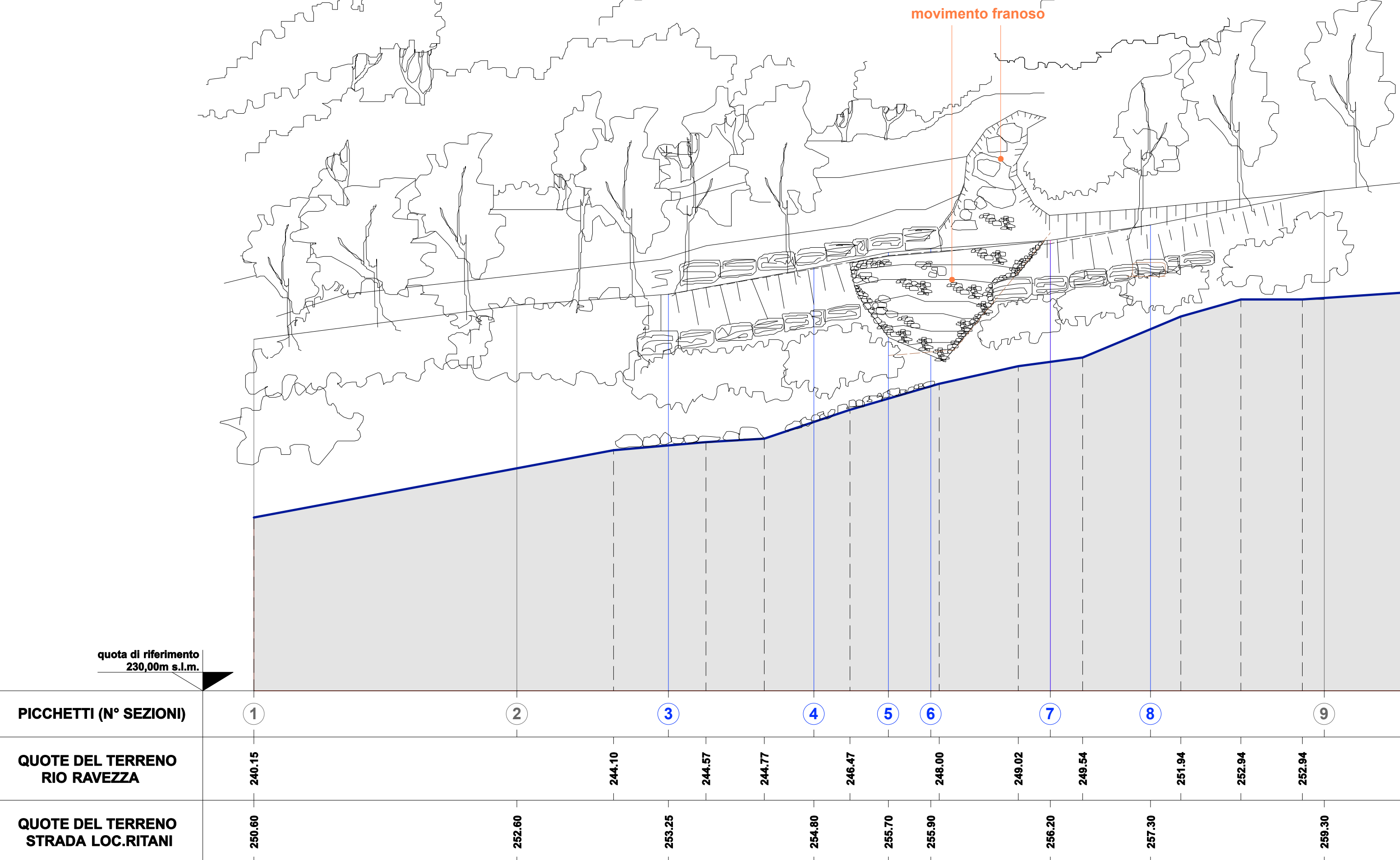
PROFILO LONGITUDINALE
