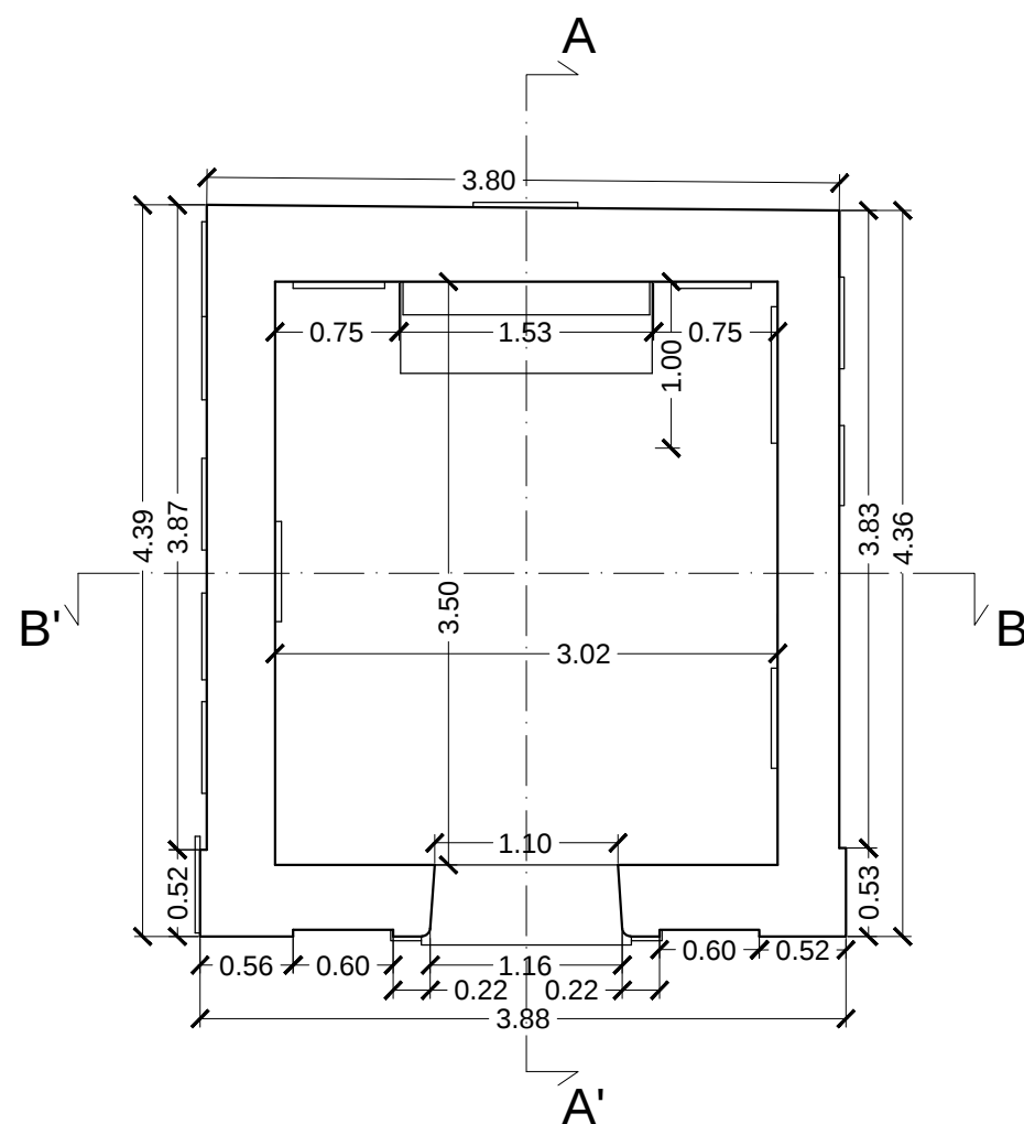
PIANTA scala 1:50
