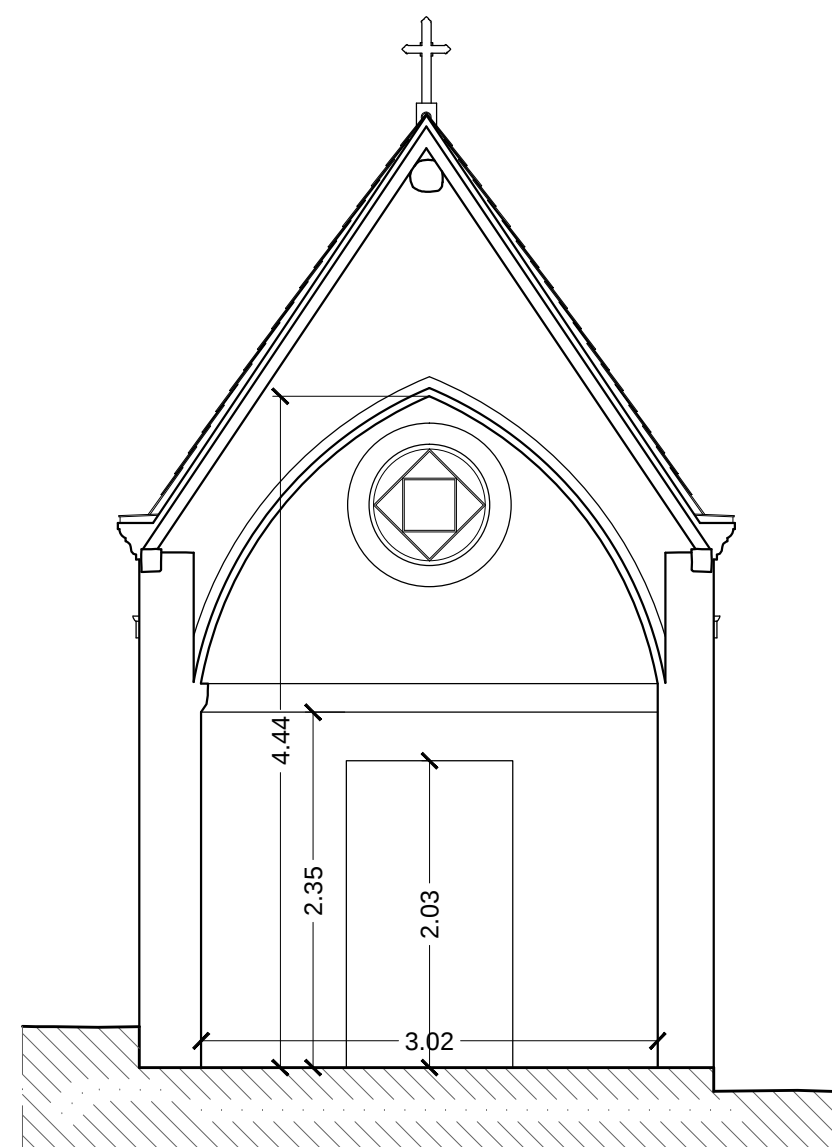
SEZIONE BB' scala 1:50
