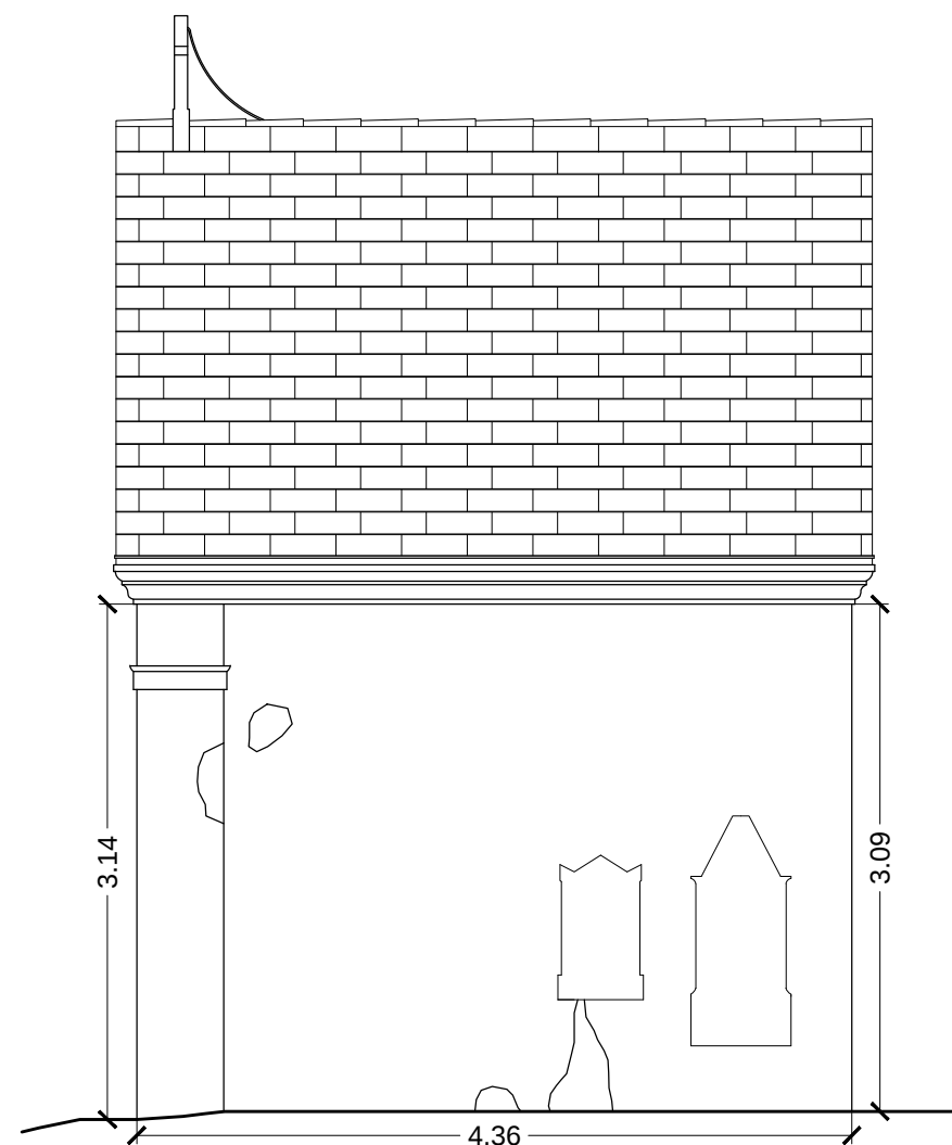
PROSPETTO EST scala 1:50
