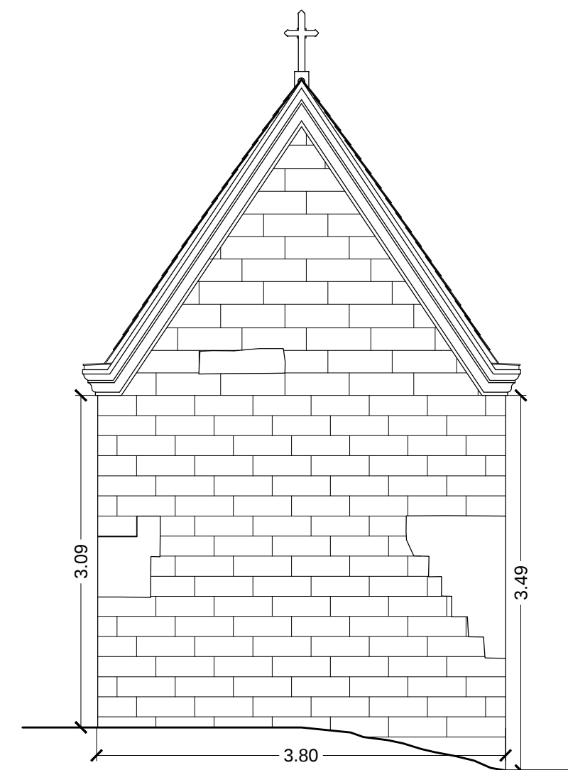
PROSPETTO NORD scala 1:50
