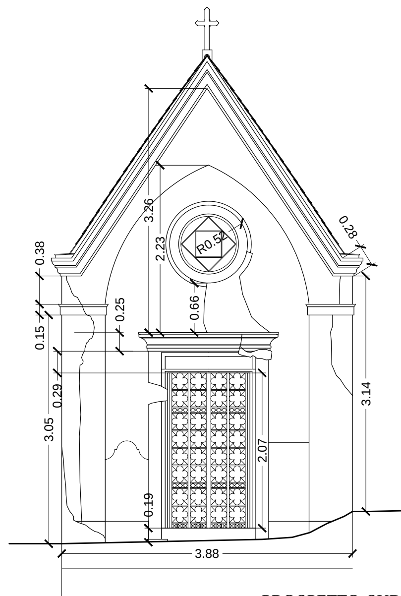
PROSPETTO SUD scala 1:50
